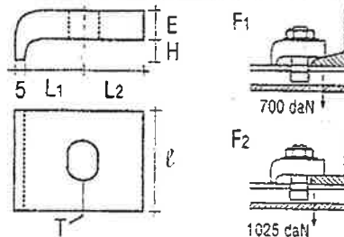
CRAPAUD DIN
